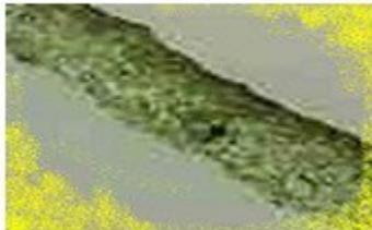
Pleurococcus viridis
